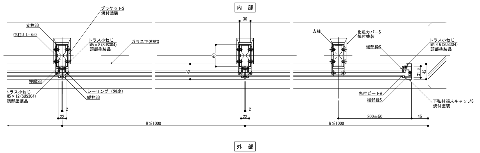
横断面図
