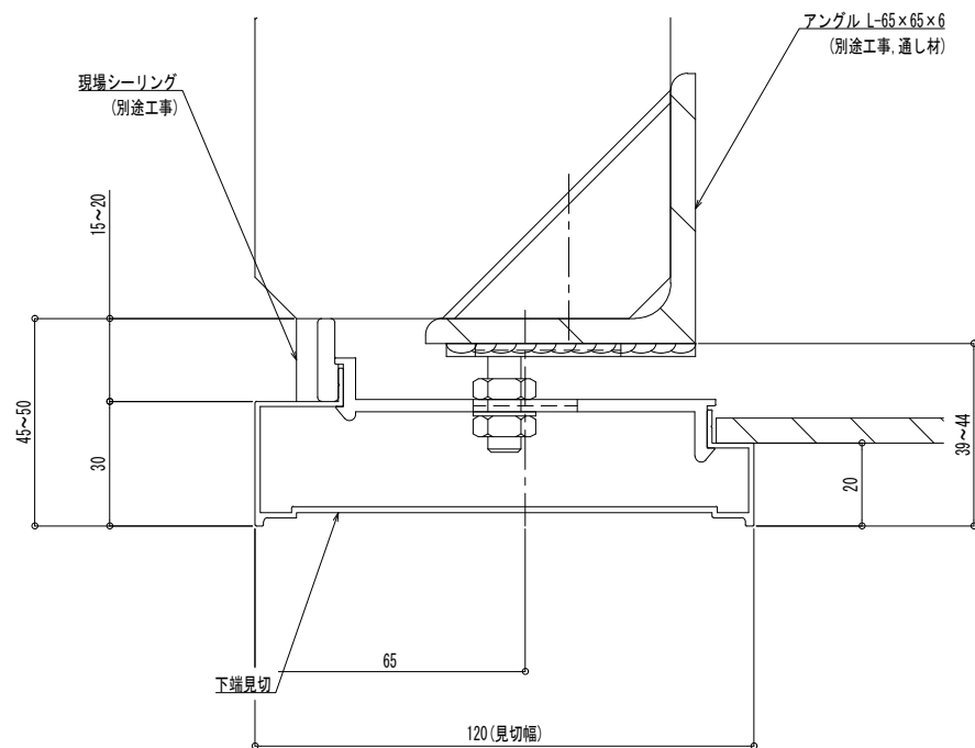
下端見切 - 120
