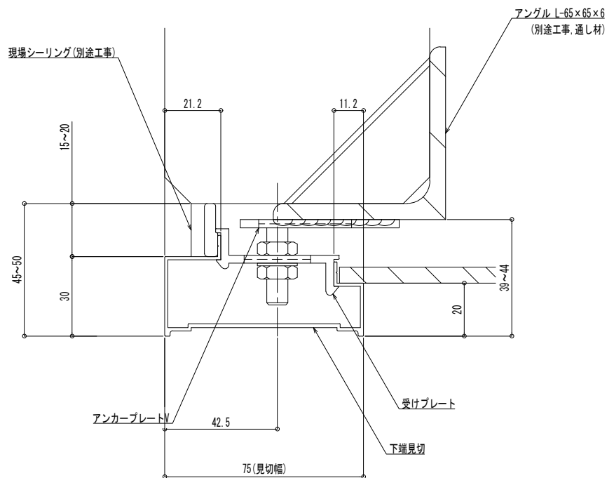
下端見切 - 75
