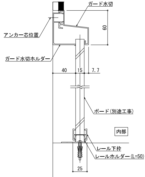
ガード水切タイプ
