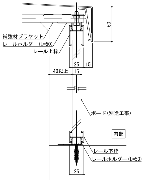
笠木・水切B
