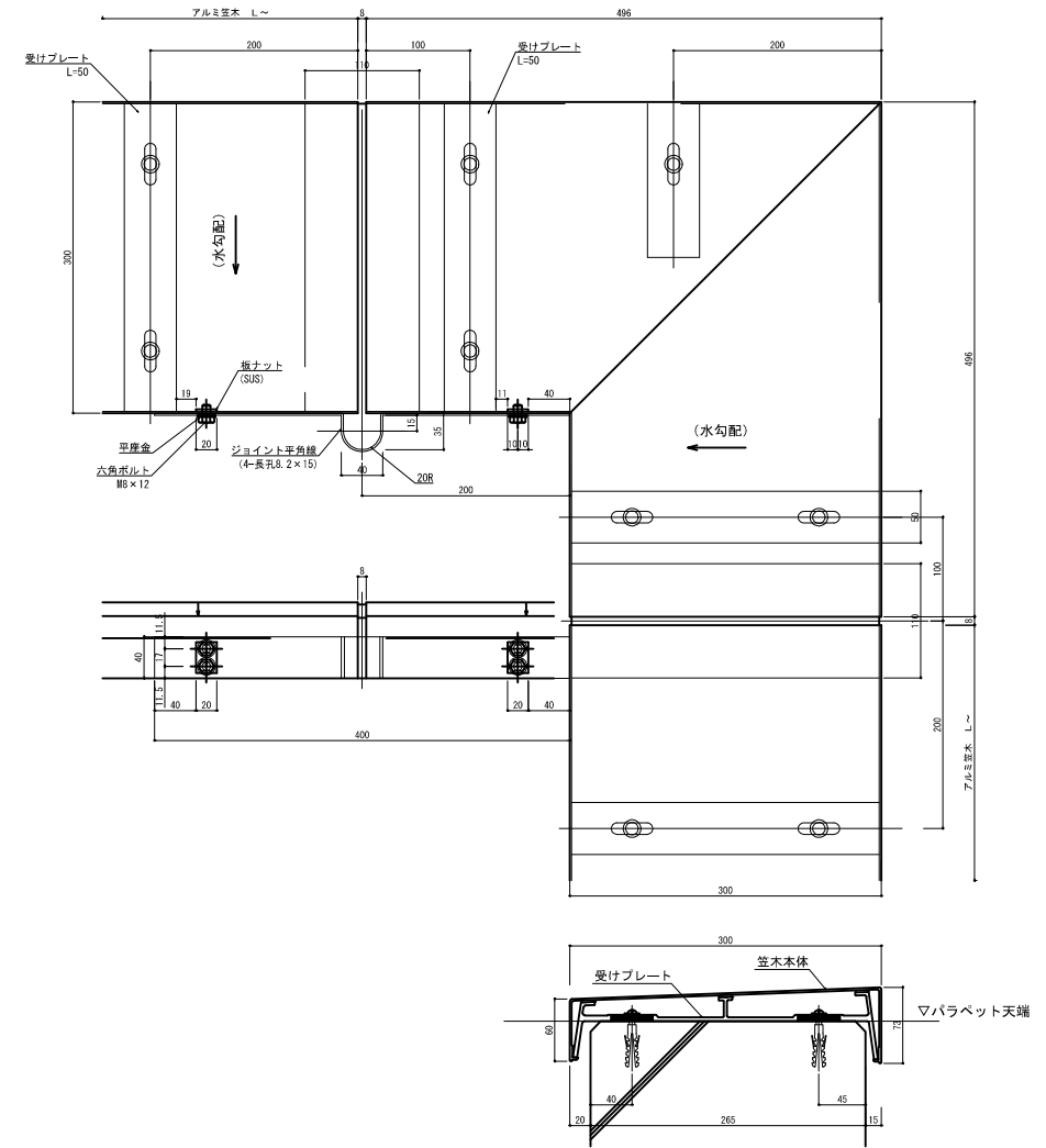
(棟上導体システム : ジョイント平角線 と 笠木コーナー 取合い図)
