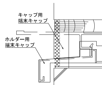
D-D断面
