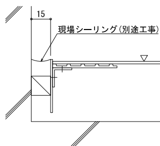
A-A断面
