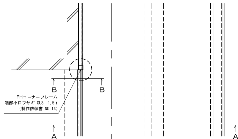
床と床コーナー取合い部平面図
