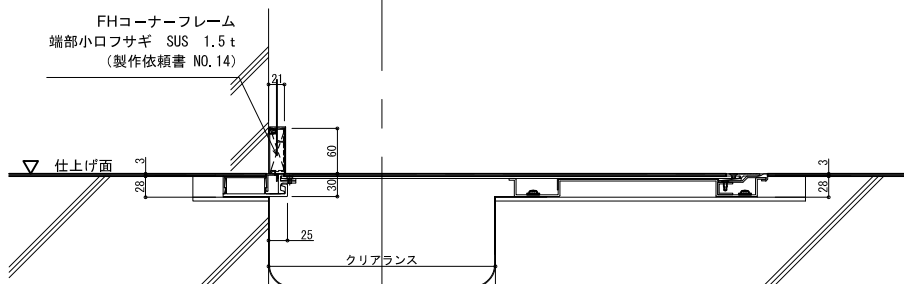
A-A 断面図
