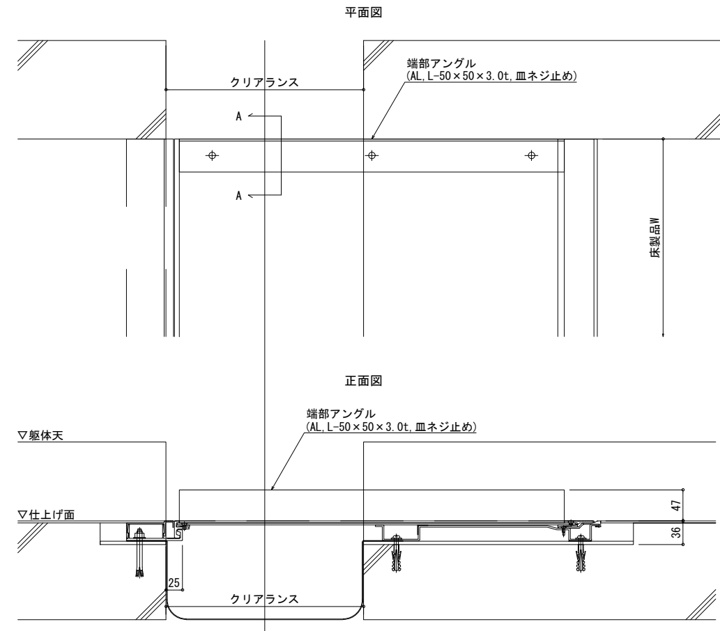
端部アングル納まり図
