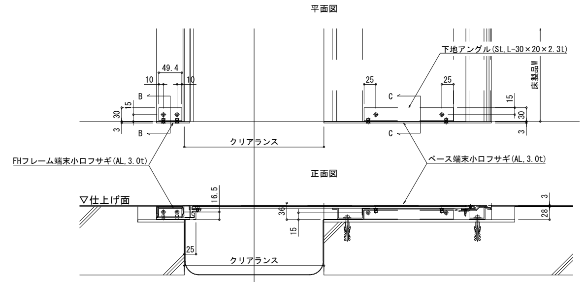
端部フサギ納まり図
