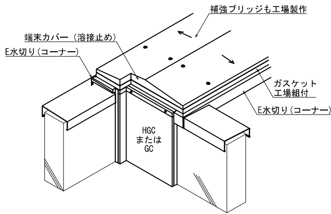
E水切りビス止め小ロフタ (AL 1.5t シルバー処理板 曲げ)
