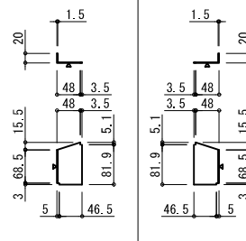
E水切りビス止め小ロフタ (AL 1.5t シルバー処理板 曲げ)
