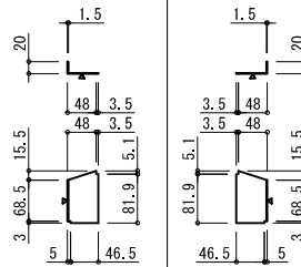
E水切りビス止め小ロフタ (AL 1.5t シルバー処理板 曲げ)
