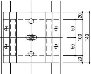
(正面立面図)
