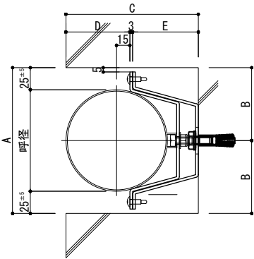
(平断面図)
