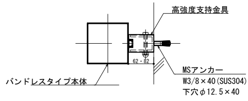
(側面図)
