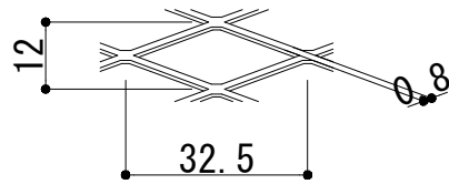
メッシュ形状
