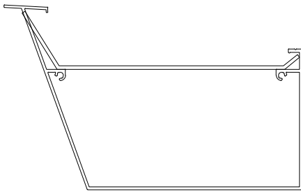
納まり図
