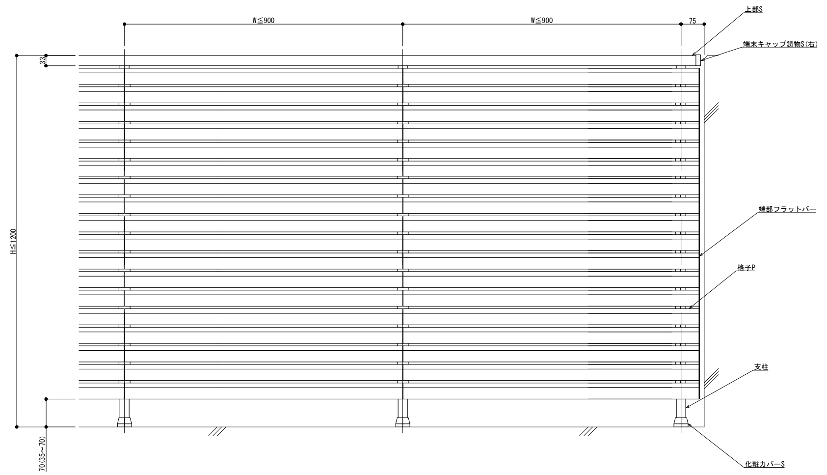
外観図
