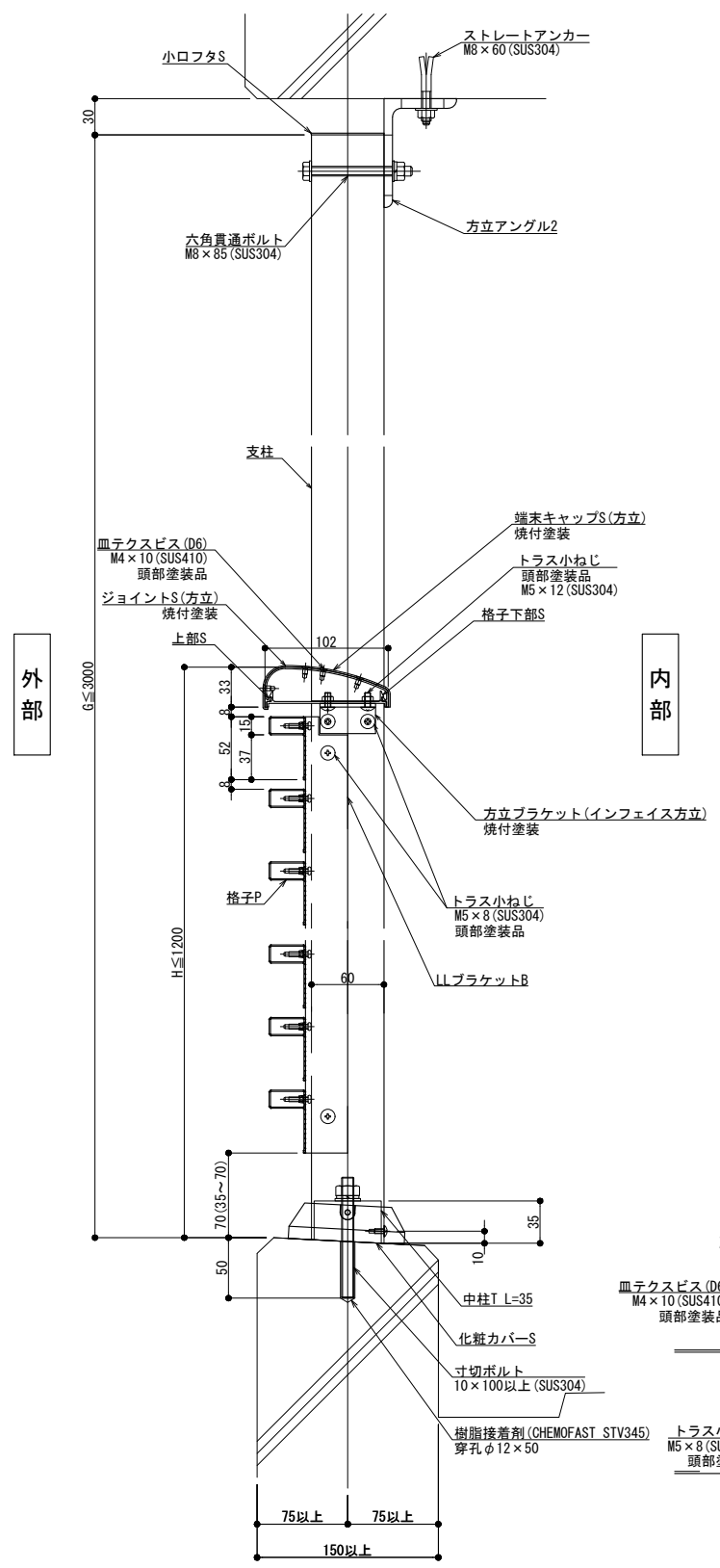
縦断面図
