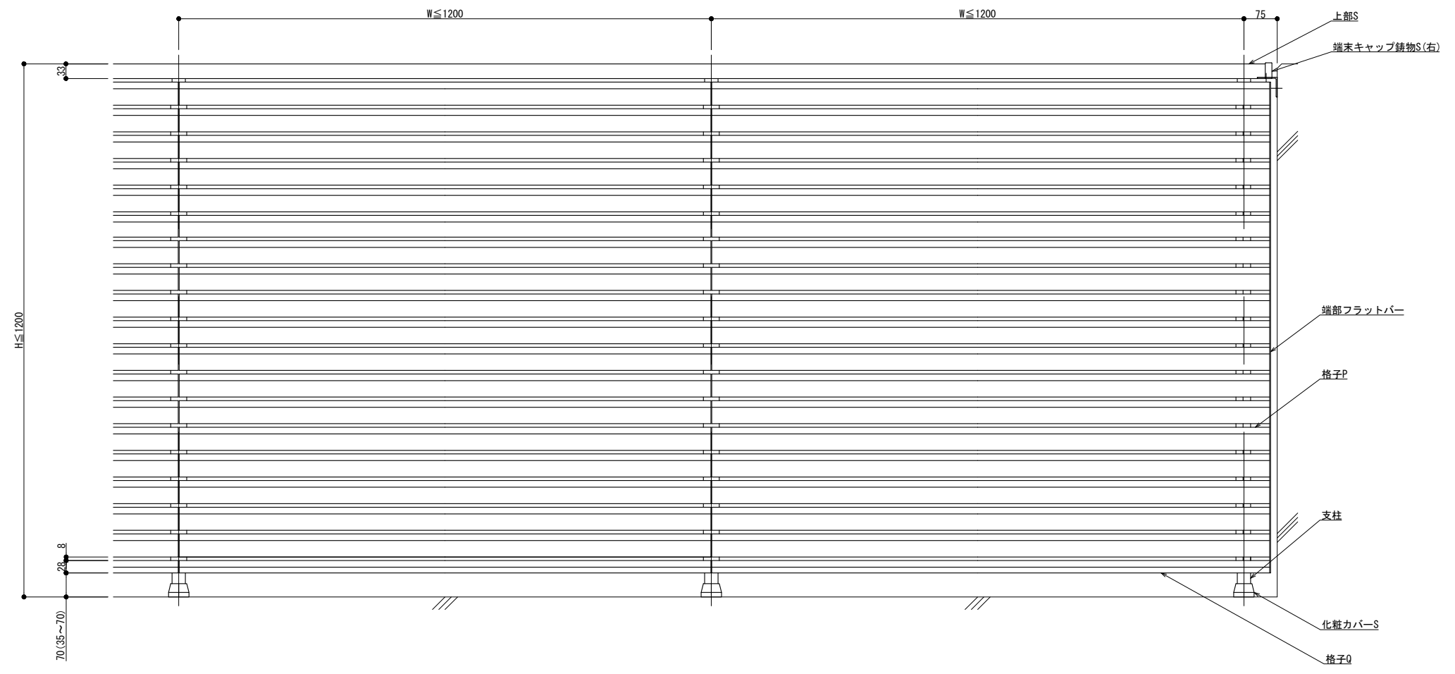
外観図
