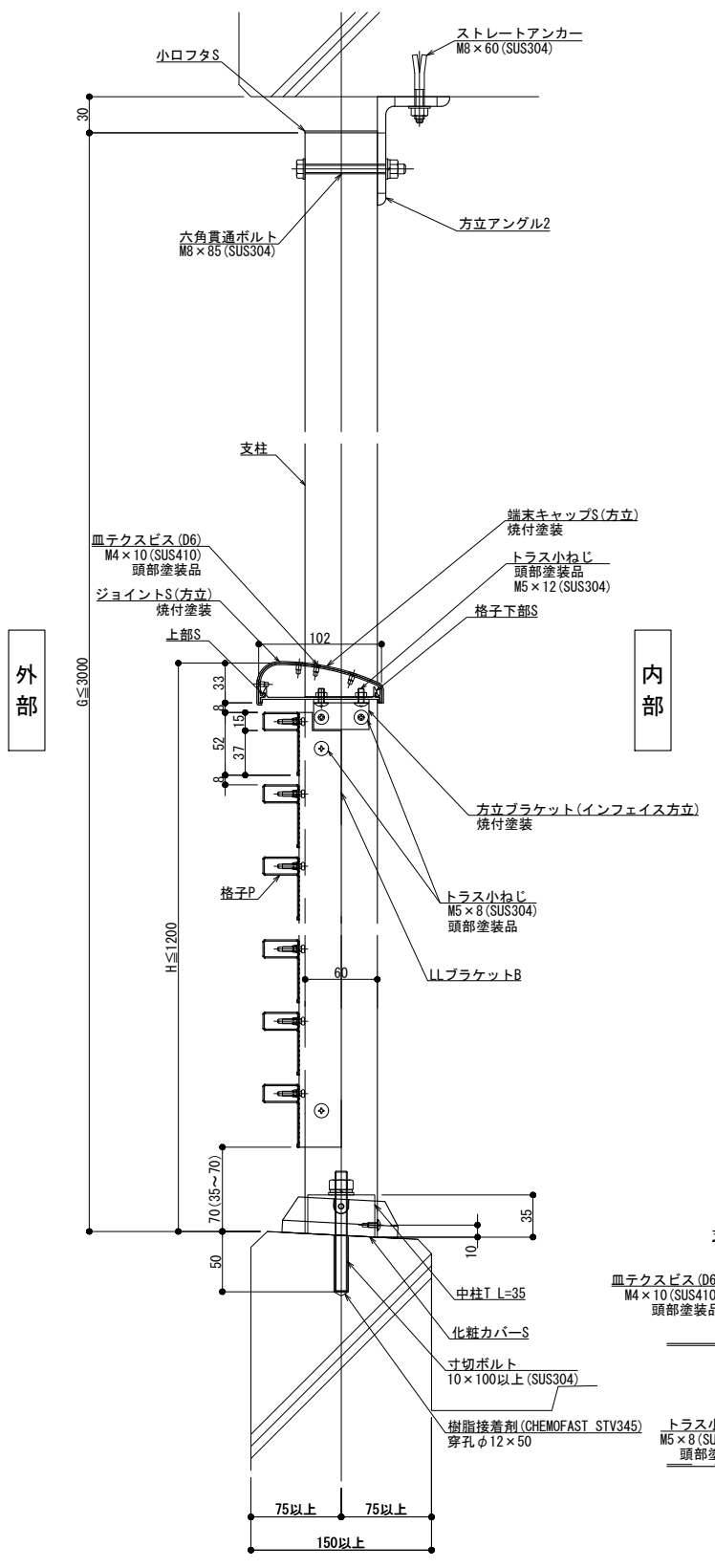
縦断面図
