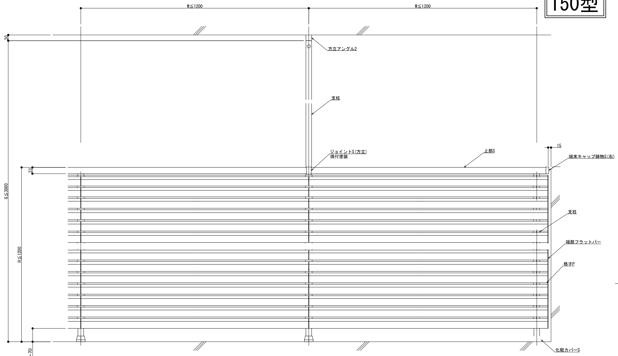
外観図
