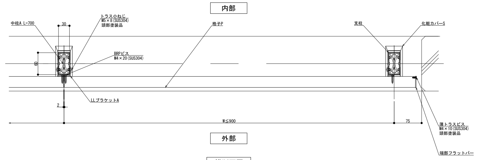
横断面図
