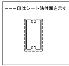
外観図 内部
