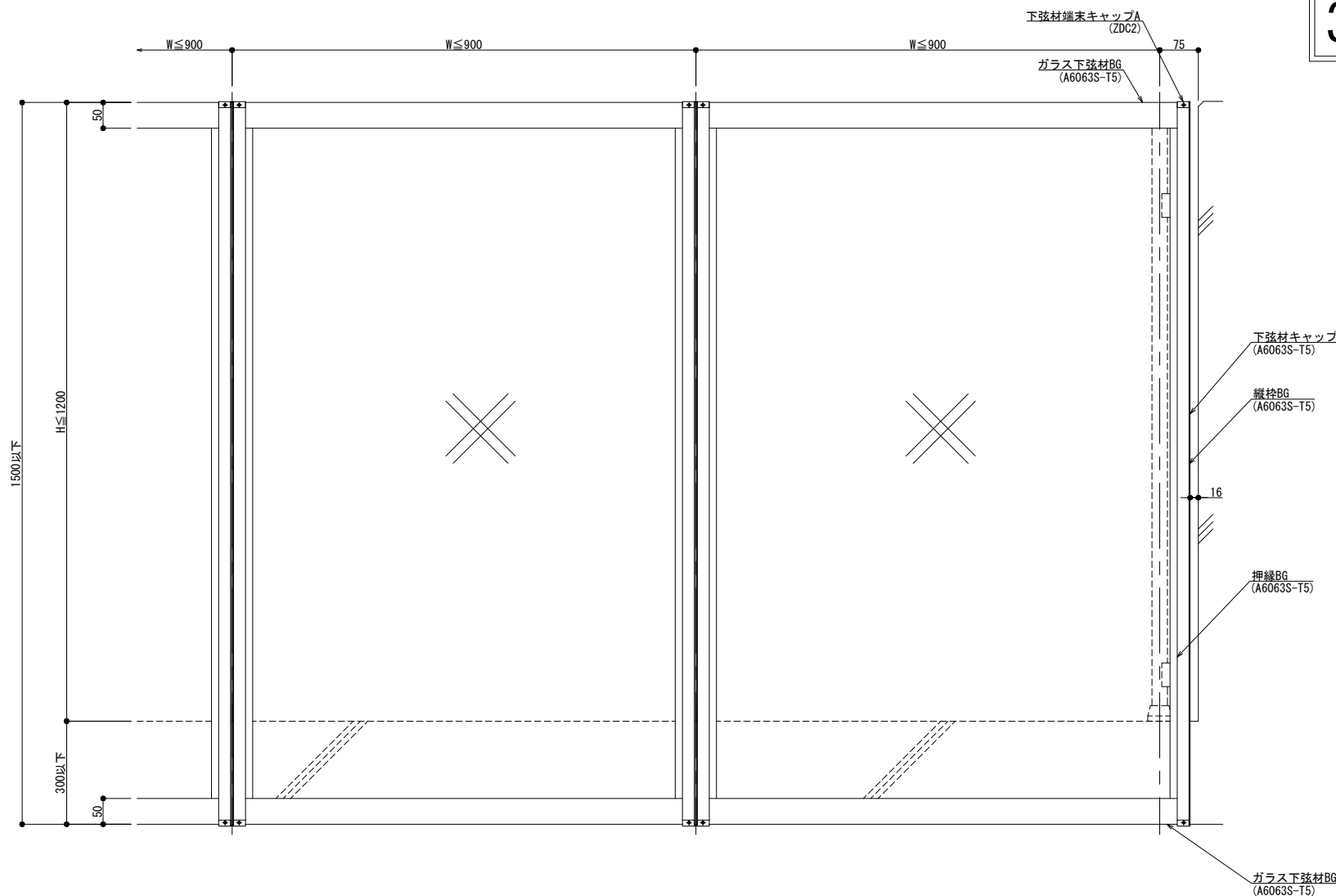
外観図
