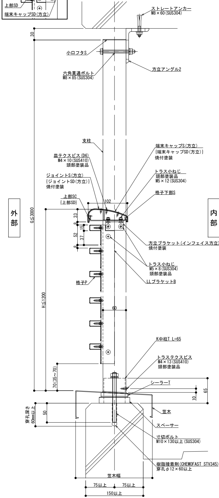
縦断面図
