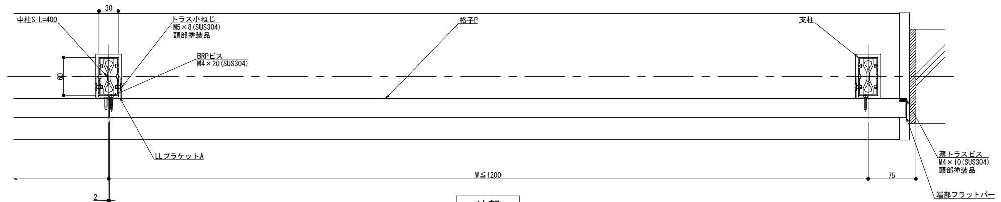
横断面図
