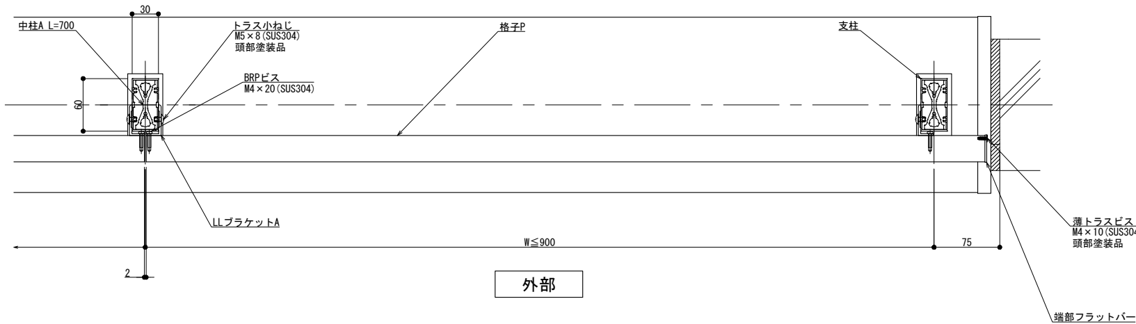
横断面図
