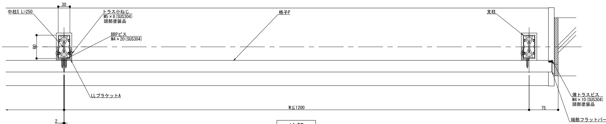
横断面図
