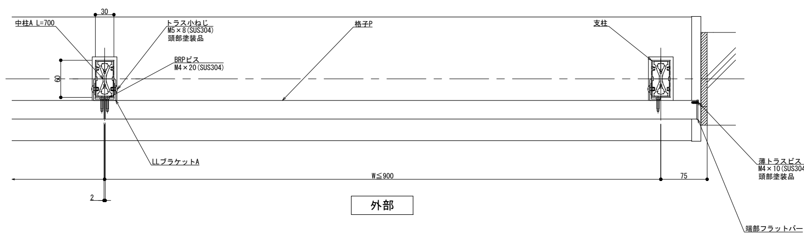
横断面
