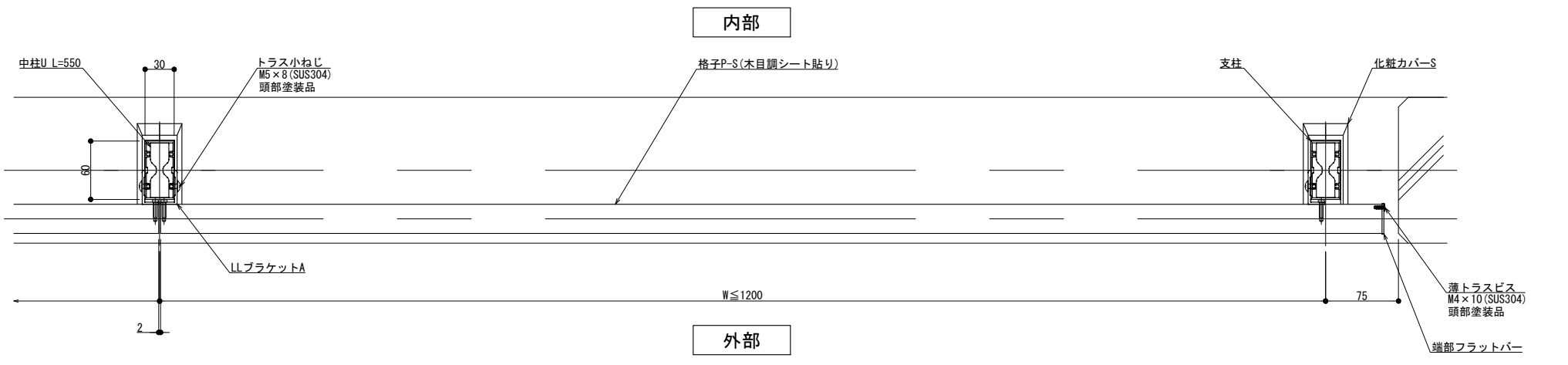
横断面図
