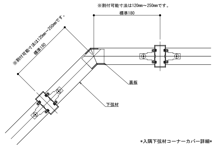
*入隅下弦材コーナーカバー詳細*
