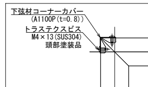
*入隅下弦材コーナーカバー詳細*
