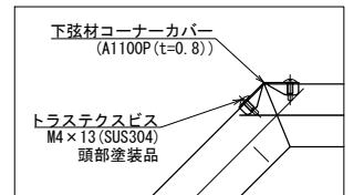
*入隅下弦材コーナーカバー詳細*
