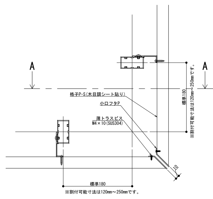
90° コーナー
