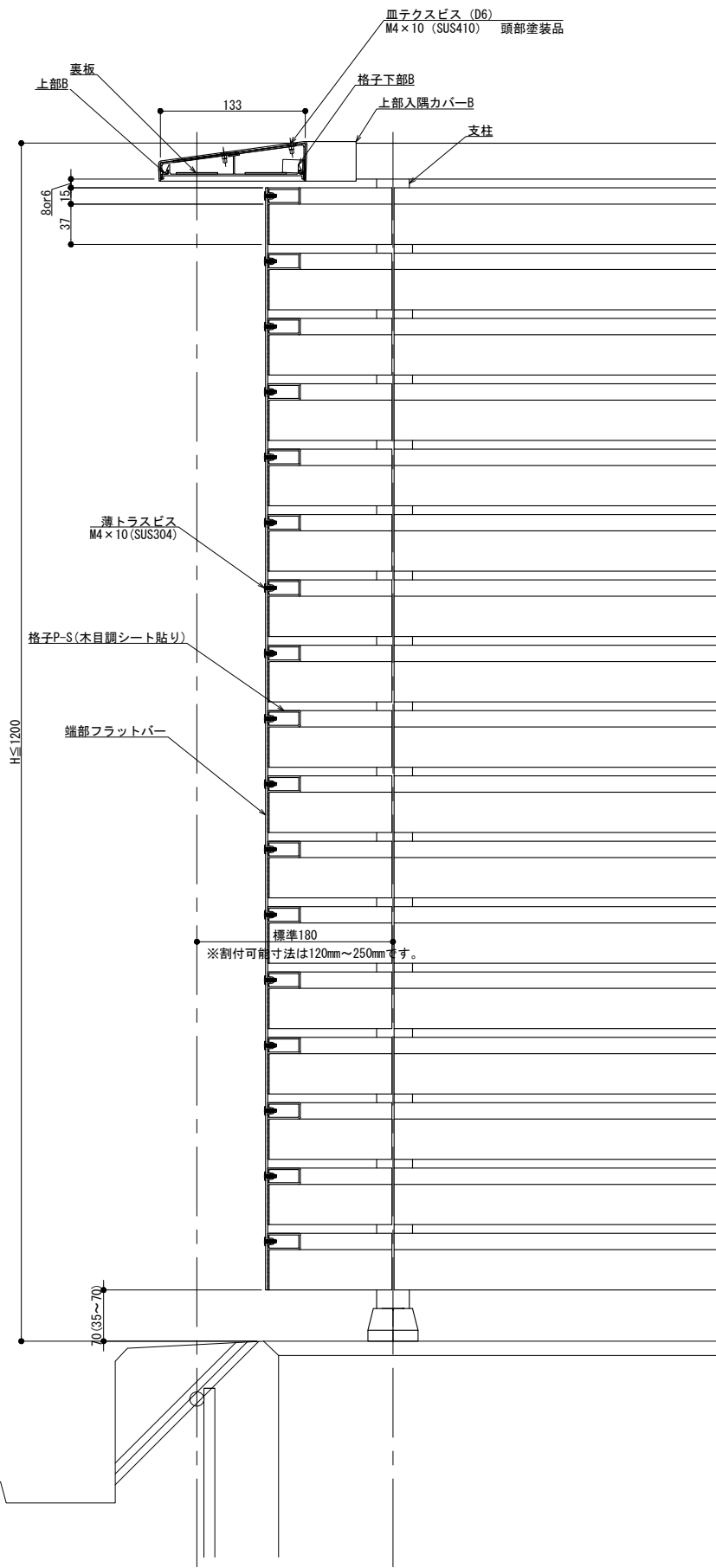
縦断面図 (A-A)
