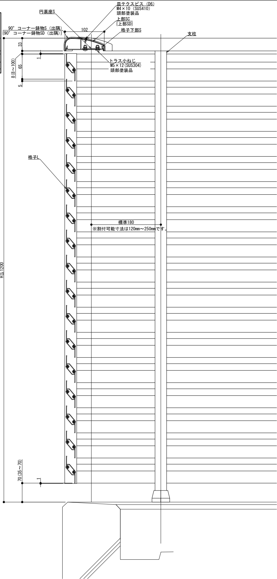
縦断面図
