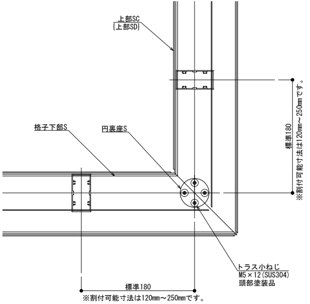
90° コーナー (格子下部S納まり)
