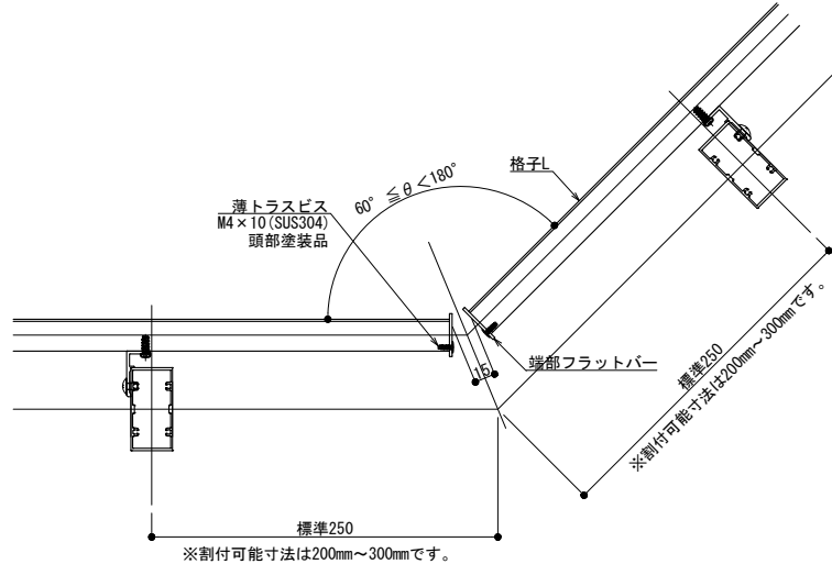
自在コーナー
