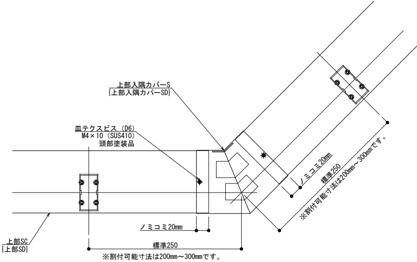
自在コーナー (上部S納まり)
