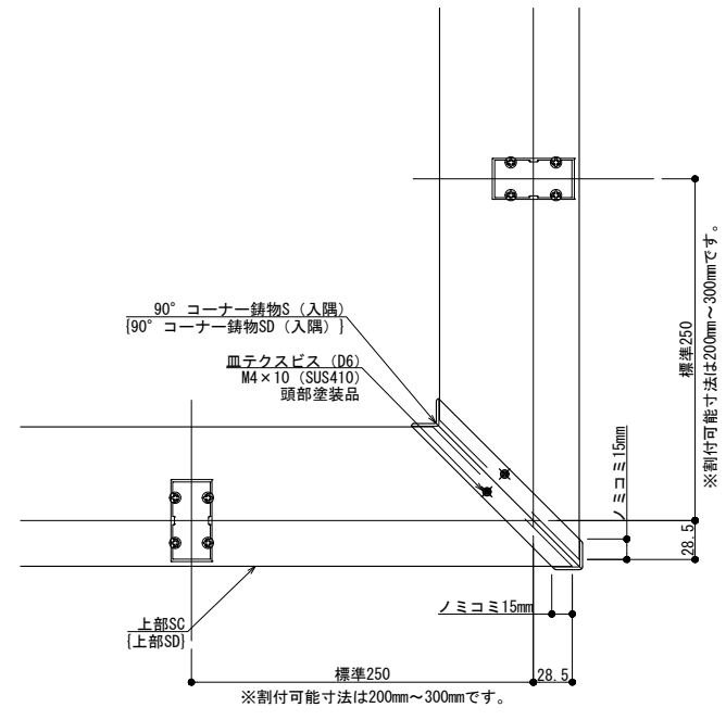
90° コーナー (上部S納まり)
