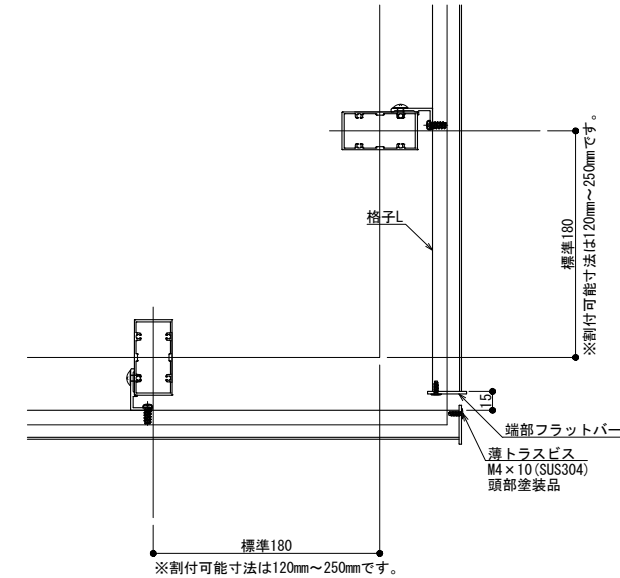
90° コーナー
