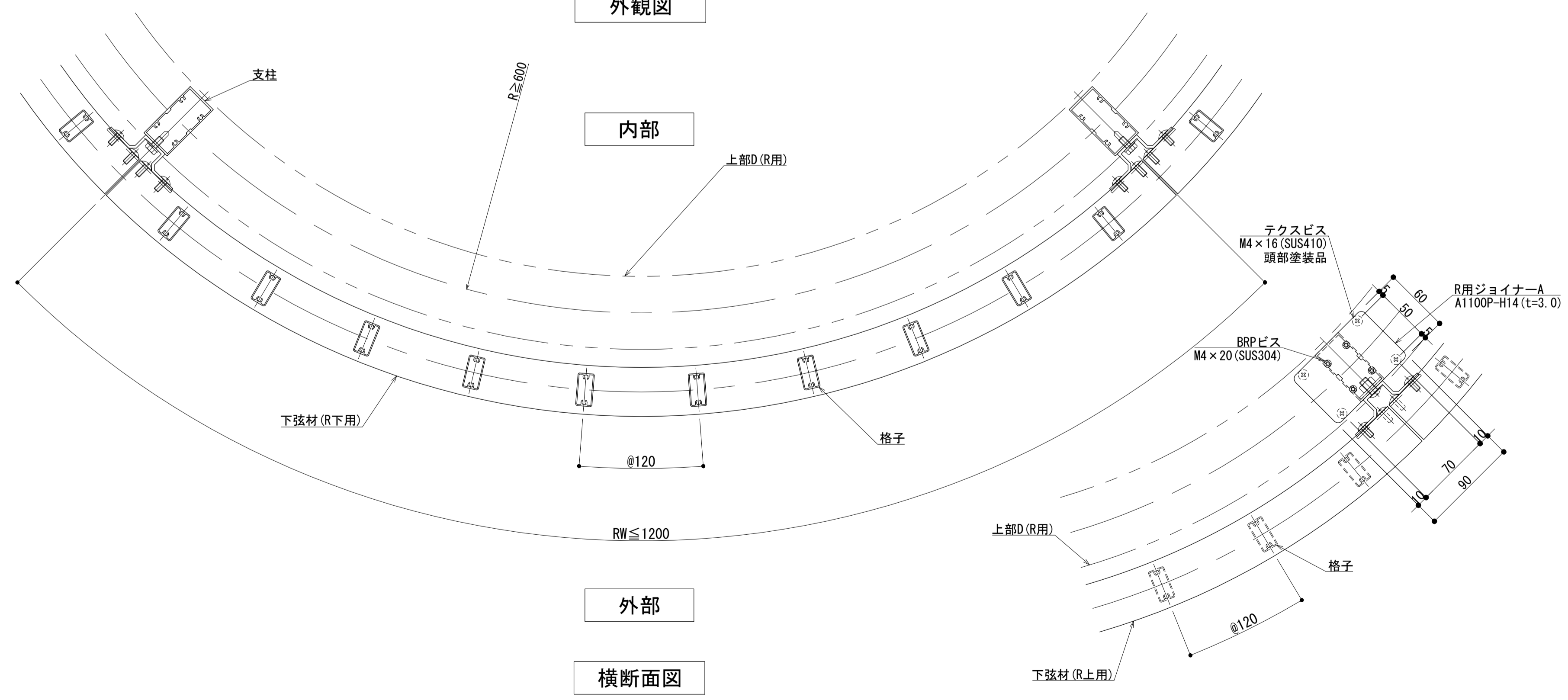
外観図
