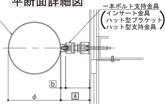
平断面詳細図
