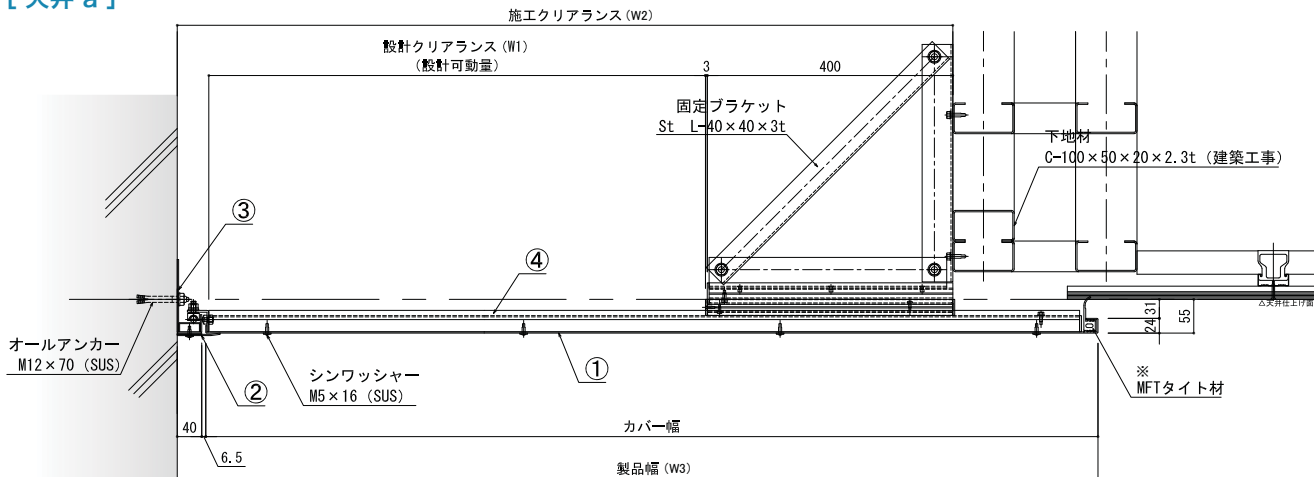
基本寸法表
