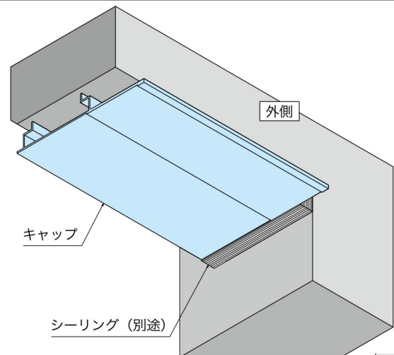
端部納まり-1
