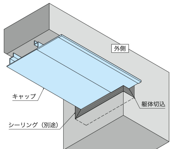
端部納まり-2
