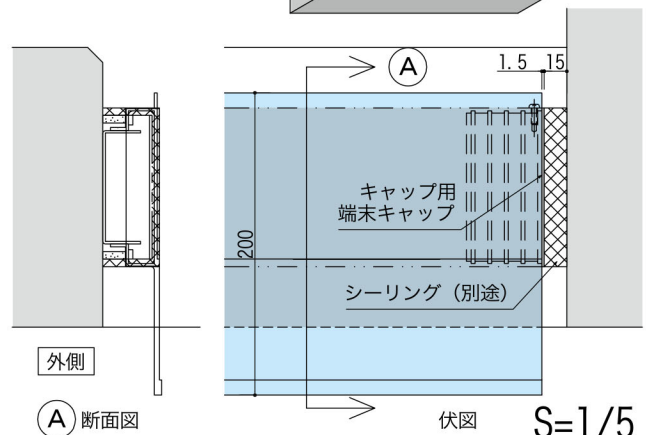
端部納まり-2
