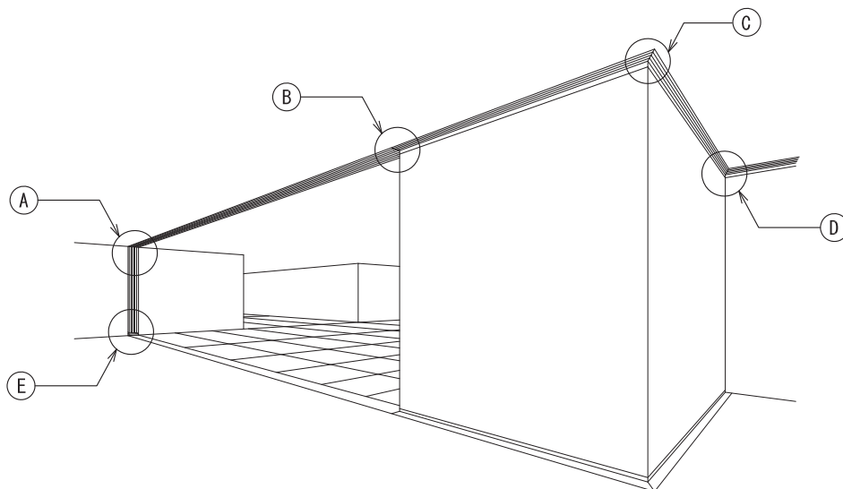
②部詳細図 S:1/5 RT-RTC 取合い部 [小口フサギ]
