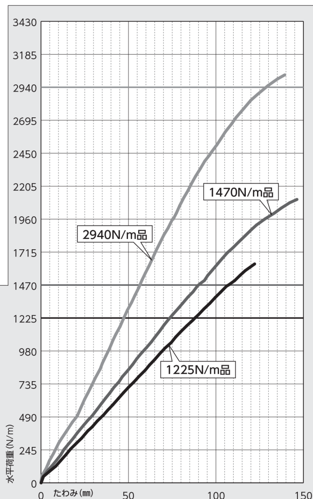
後付工法試験結果
