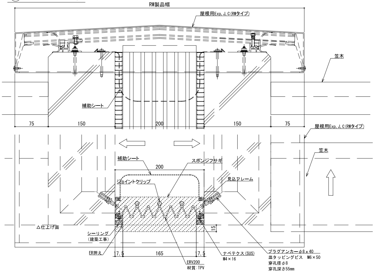
Ⓐ 部詳細図 S:1/5
