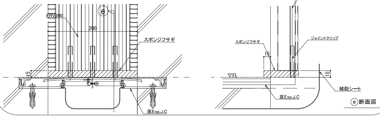
⑤部詳細図 S:1/5
