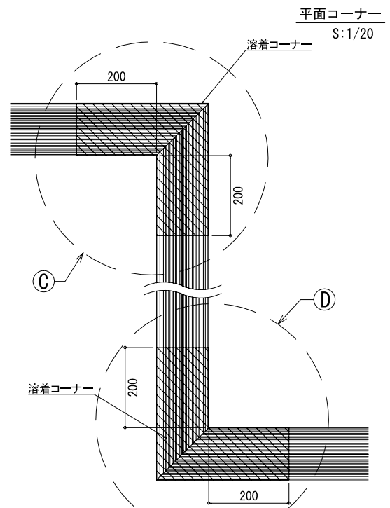
③部詳細図 天井コーナー(出隅) ④部詳細図 天井コーナー(入隅)
