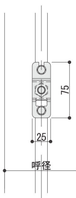
B-B断面詳細図
