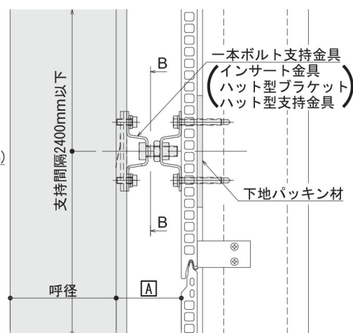
立面図
